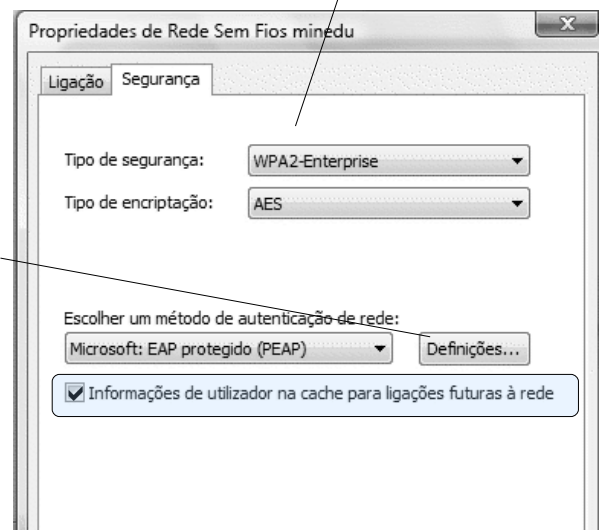
Figura 8: Definir Segurança
