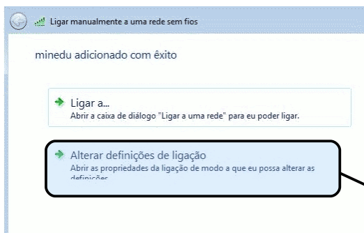
Figura 7: Alterar definições...
