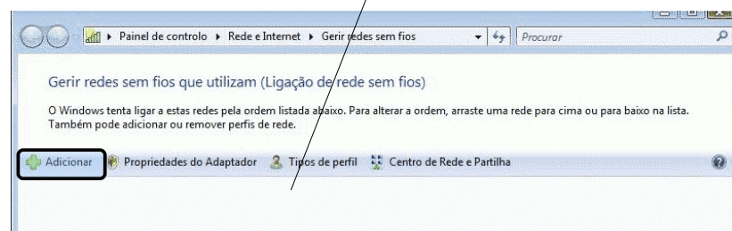
Figura 4: Seleccionar Adicionar
