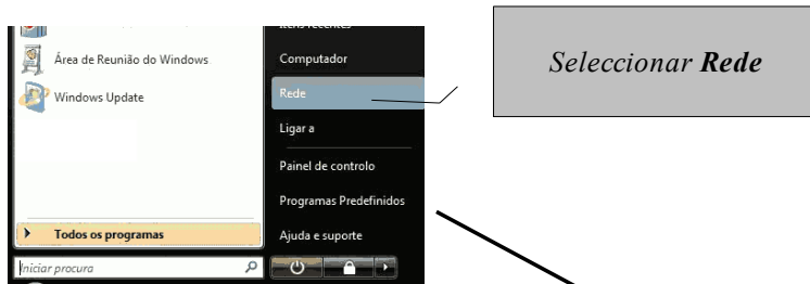
Figura 1: Menu Iniciar
