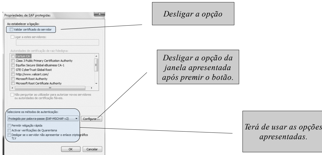
Figura 9: Definir EAP
